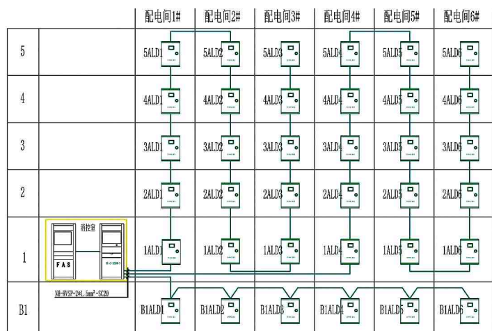
应急照明系统干线图
