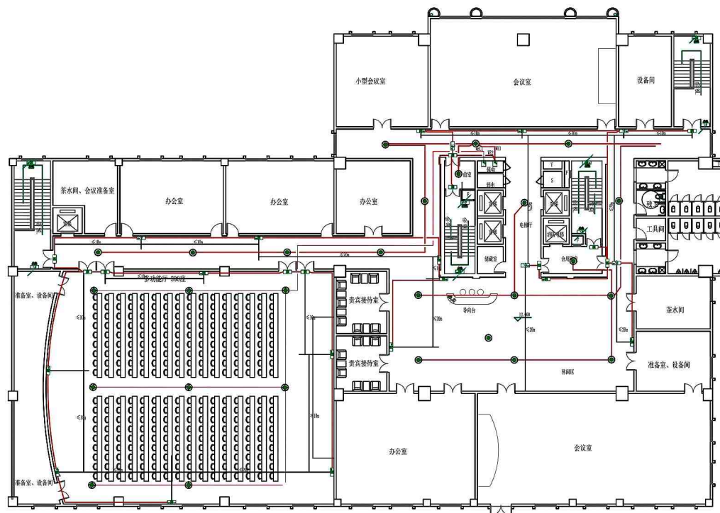
应急照明系统平面图
